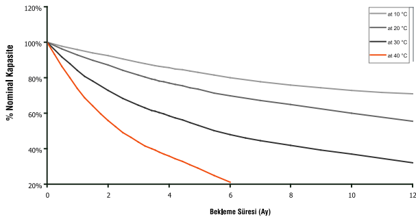
Kendi kendine deşarj
