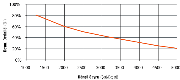
Döngü Sayısı-Deşarj Derinliği
